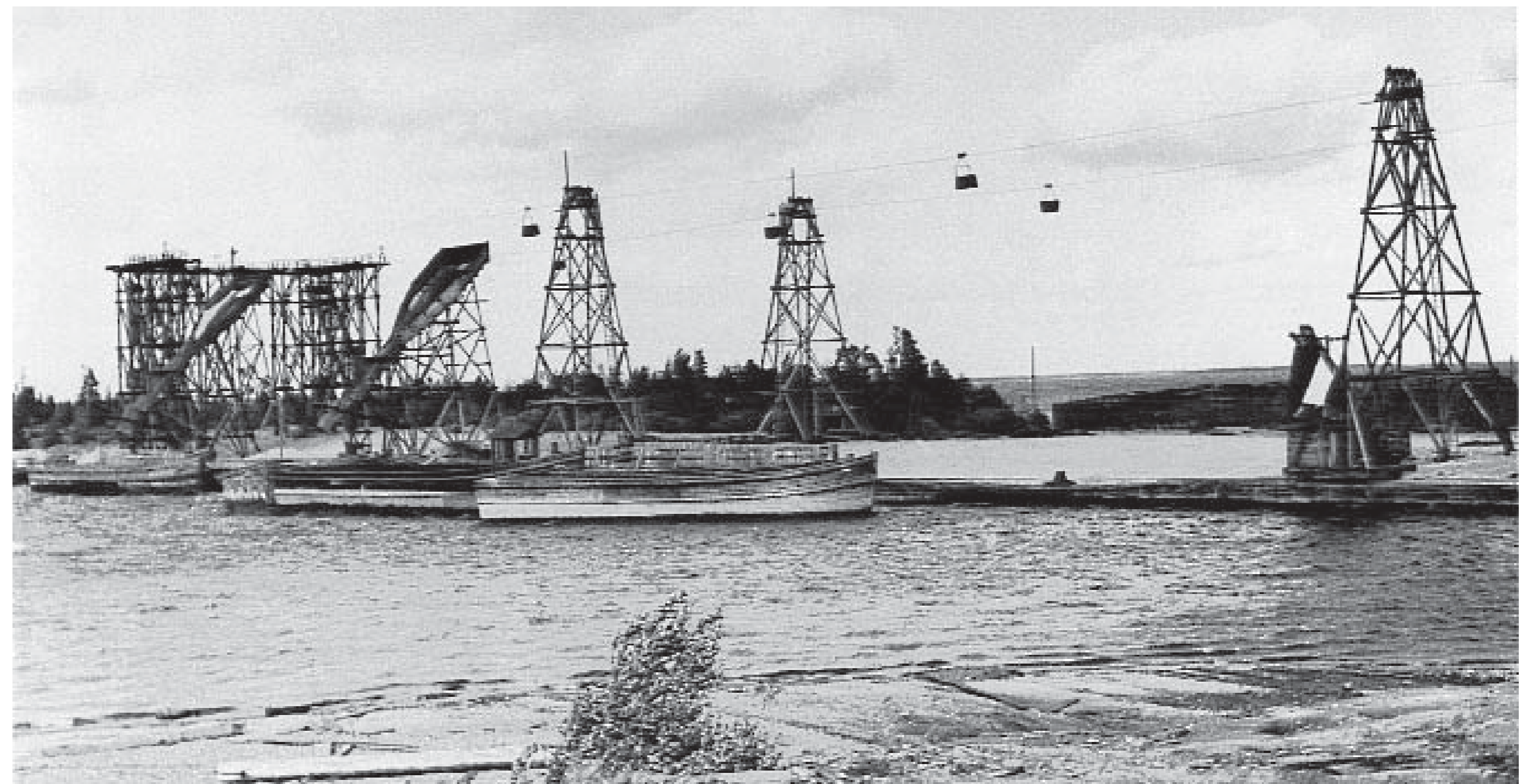
Linbanan och spånlastningen
